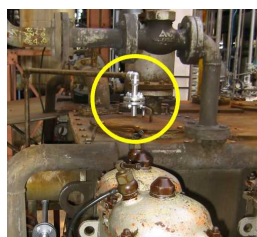
↑ 返油用配管 オイルタンクのフタ にフランジを溶接 ← メッシュフィルター (洗浄再生式)
